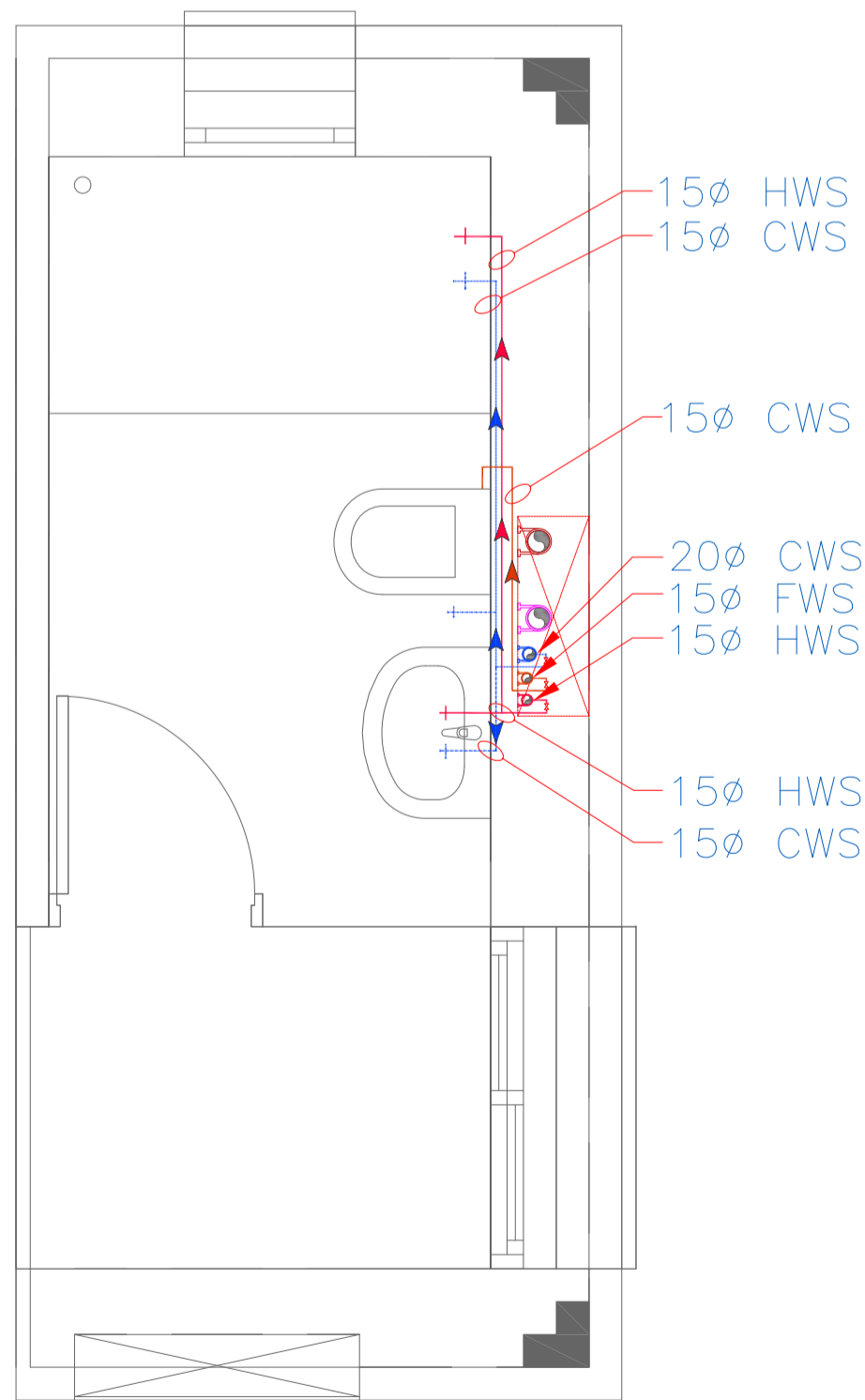
3 Toilet - 1 : Water Supply Layout Scale : 1:25
