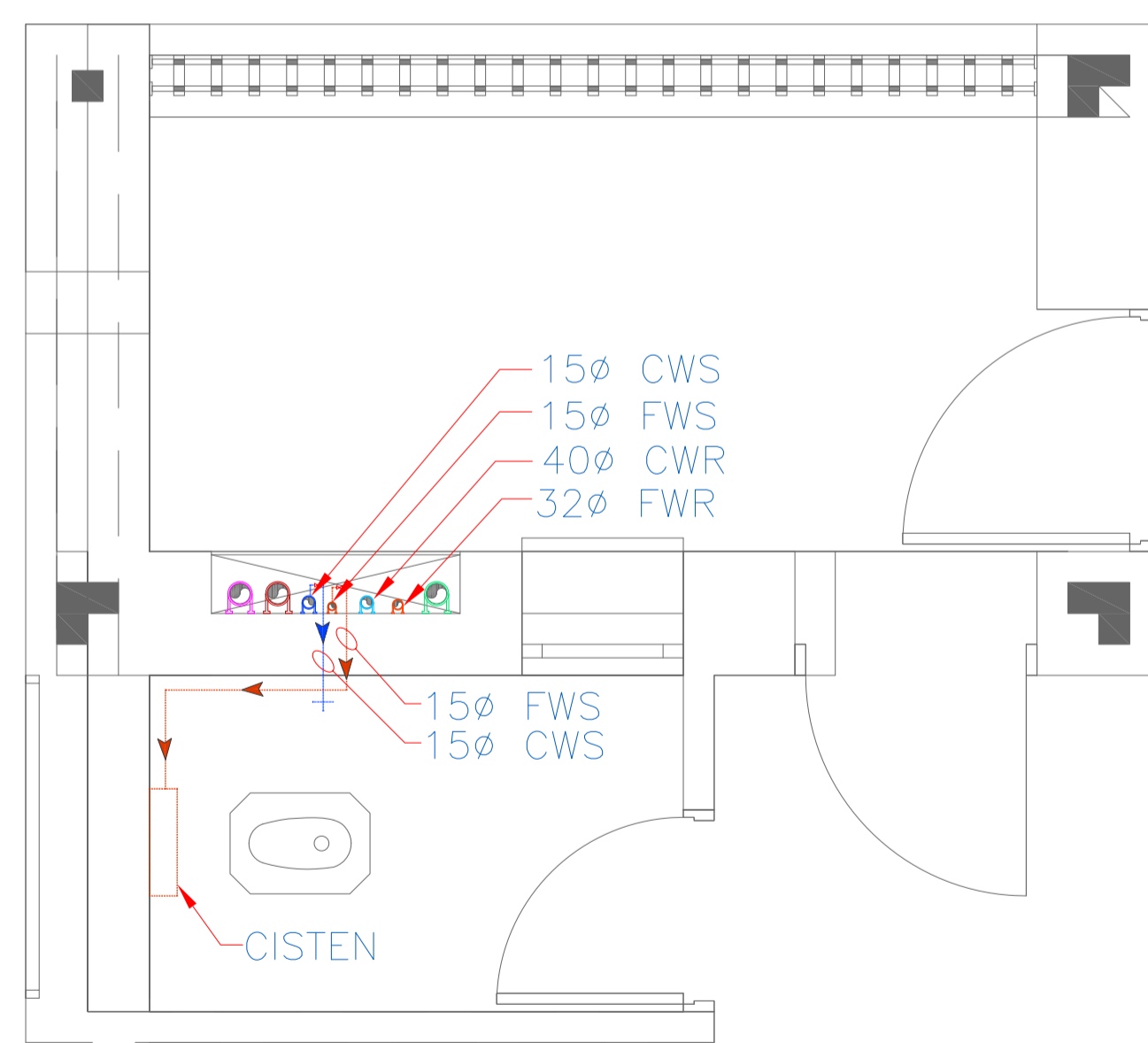
2 Toilet - 2 : Water Supply Layout Scale : 1:25
