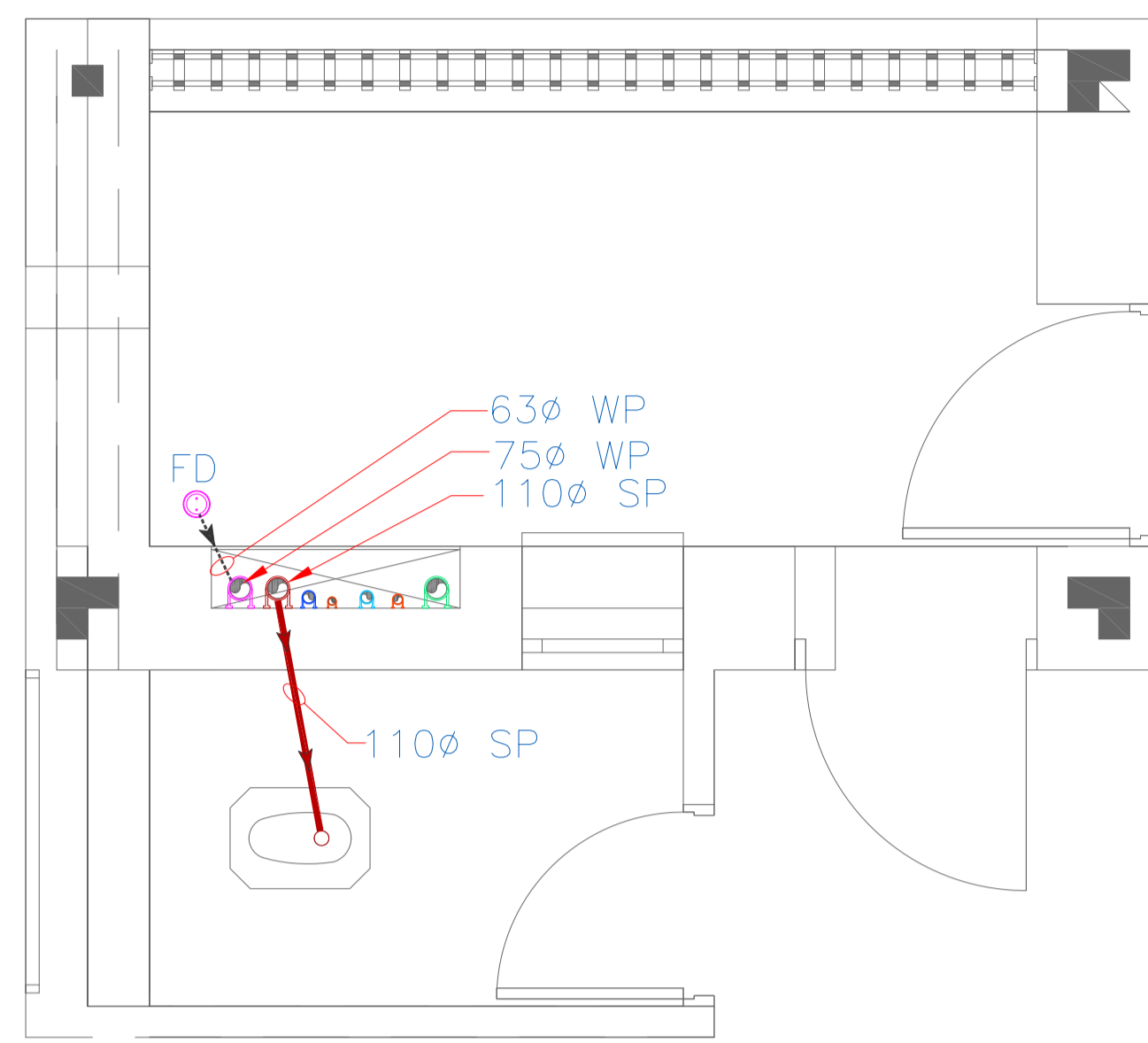
5 Toilet - 2 : Drainage Layout Scale : 1:25
