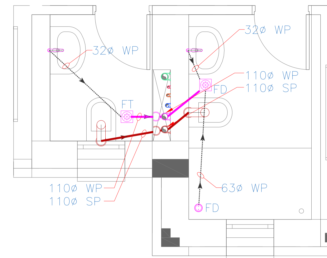
4 Toilet - 3 : Drainage Layout Scale : 1:25
