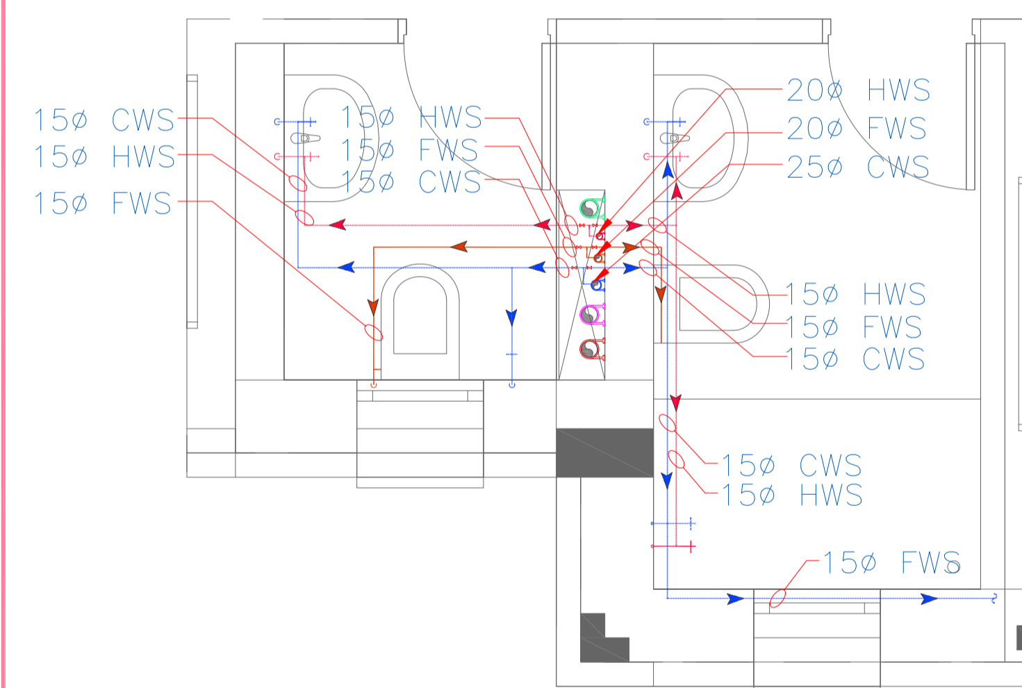
1 Toilet - 3 : Water Supply Layout Scale : 1:25
