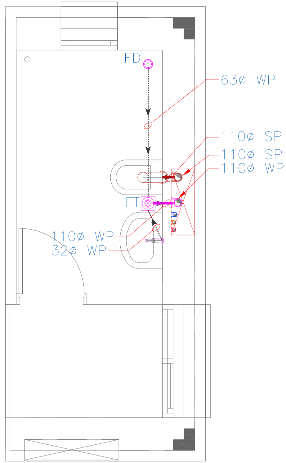
6 Toilet - 1 : Drainage Layout Scale : 1:25
